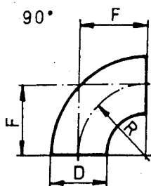
OBLOUKY
