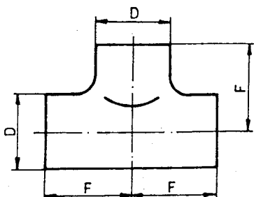
TVAROVKY T
